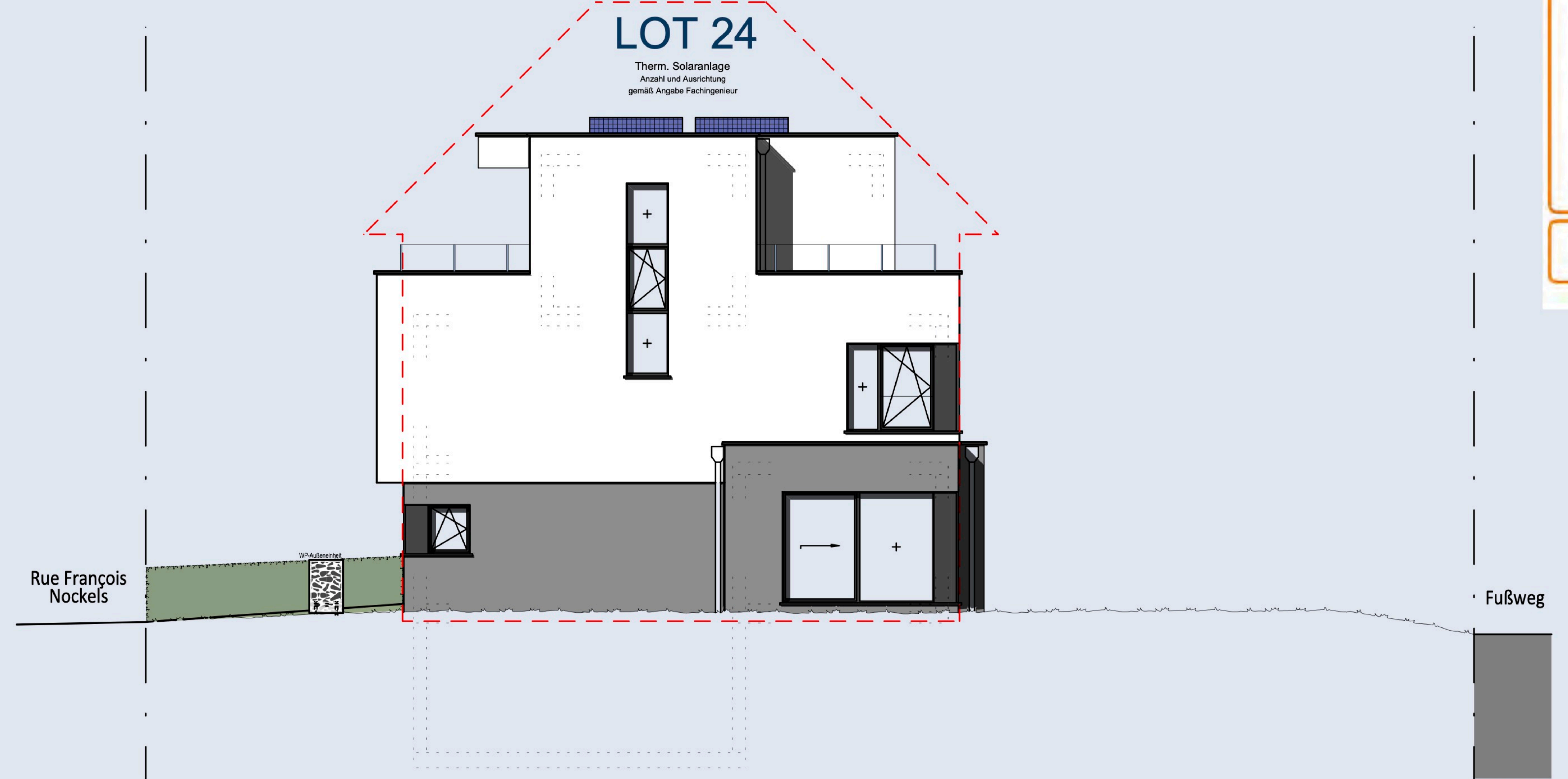
ANSICHT RECHTS
