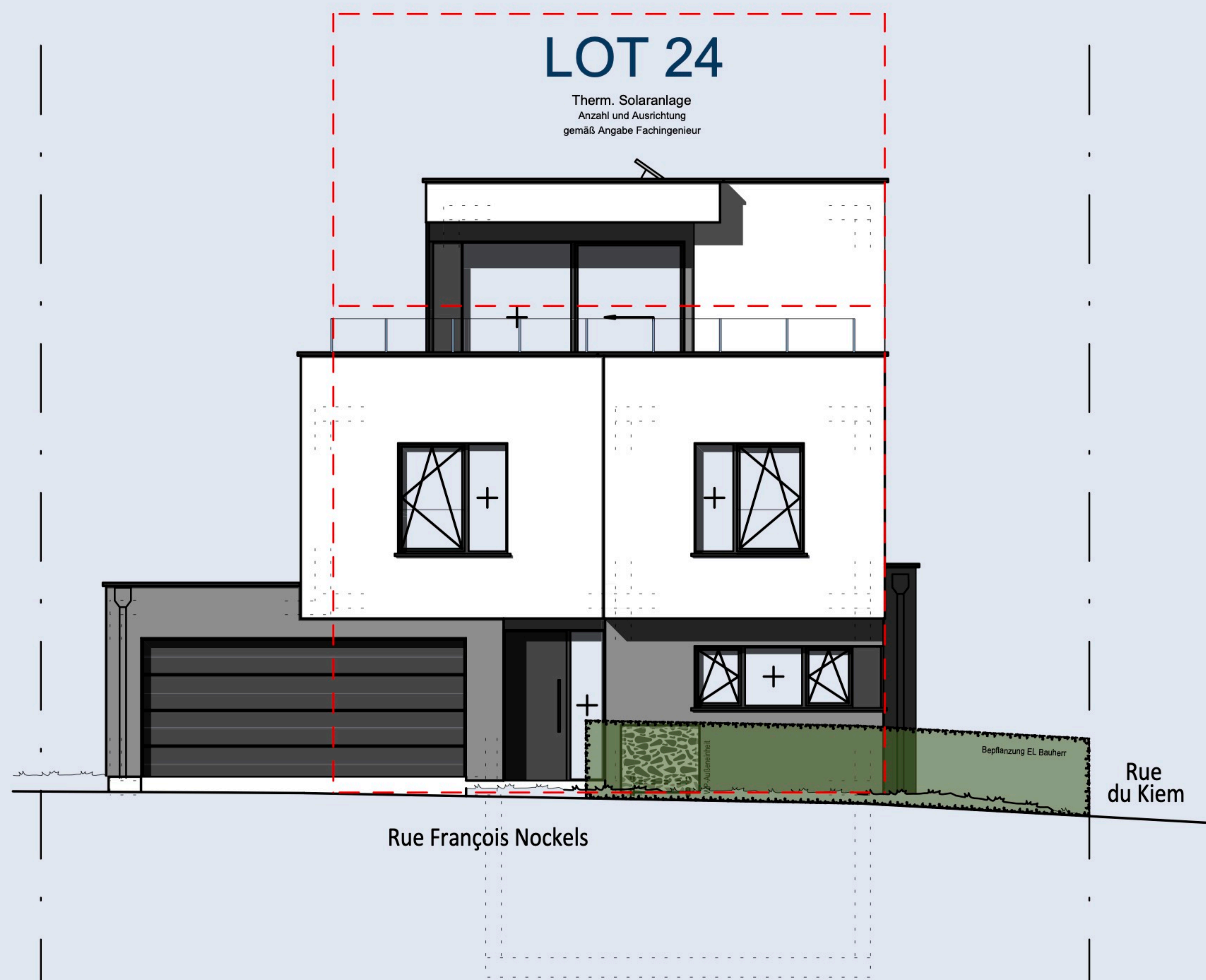
ANSICHT STRASSE
