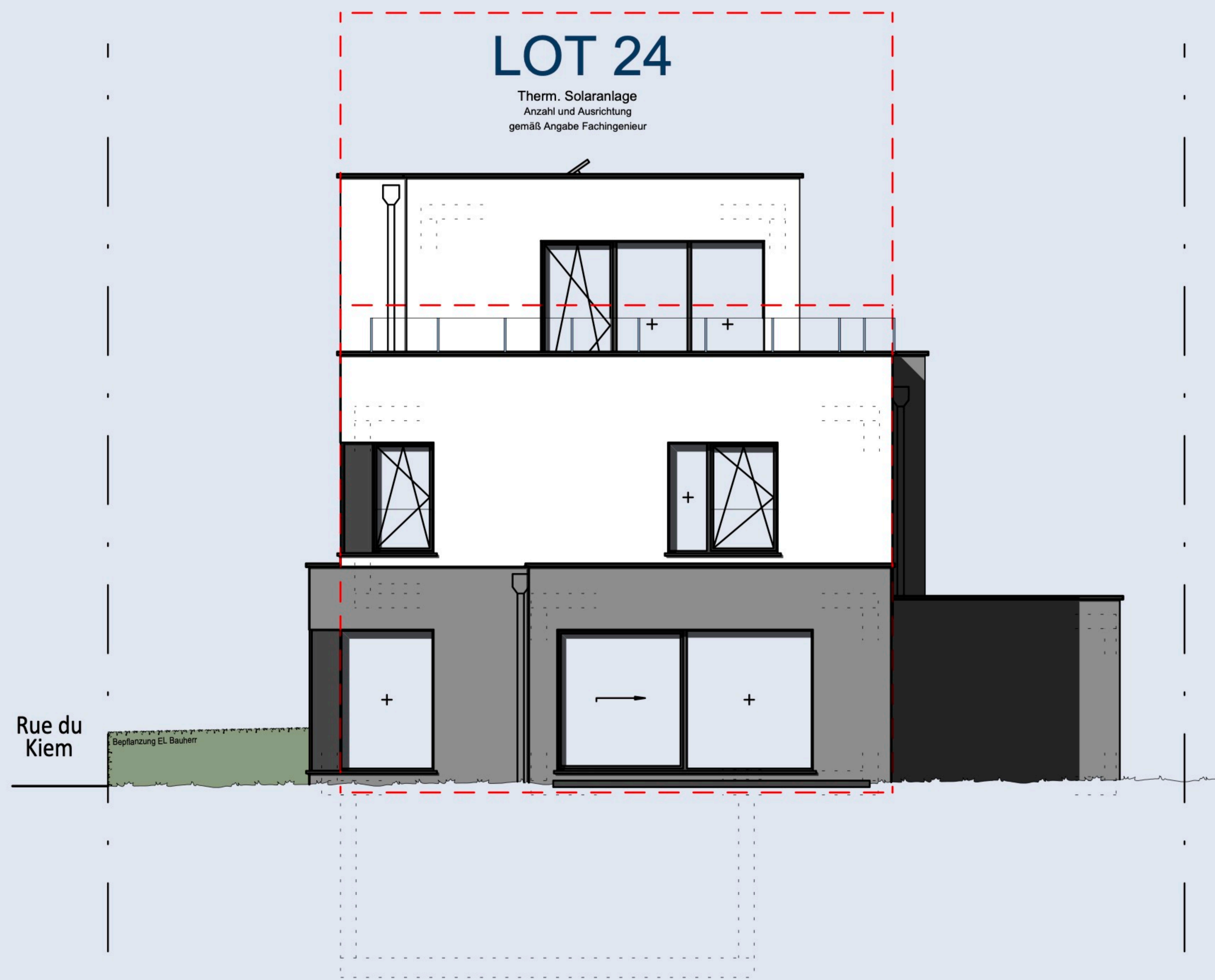
ANSICHT GARTEN
